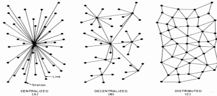
Şekil 1: Ağ Tipleri
